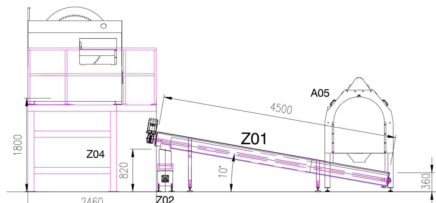
VIEW A-A
